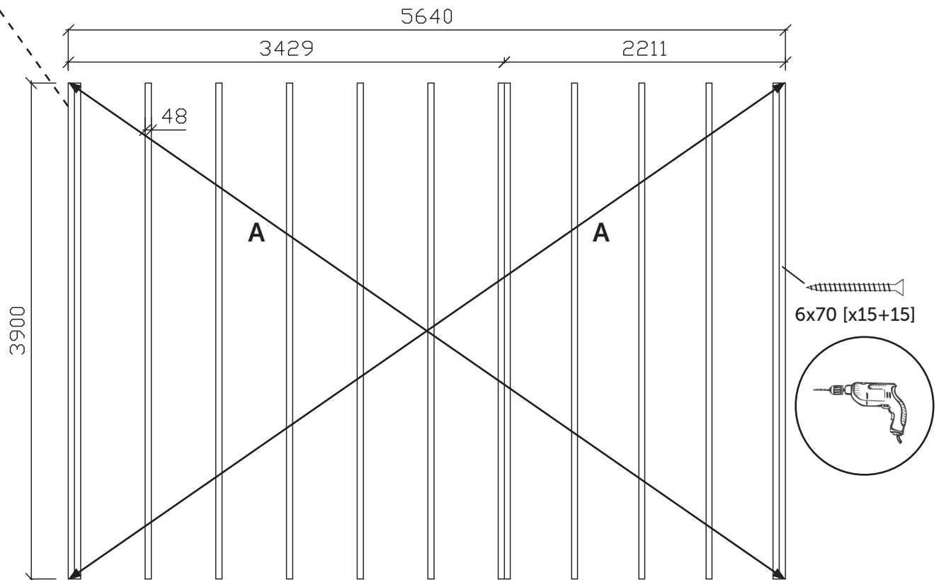
Perustuspuiden asettelu - Monteringen av grundbalkarna Monteringen av grunnbjelkene - Monteringen af fundamentbjælkerne Assembling of foundation beams - La pose des solives
