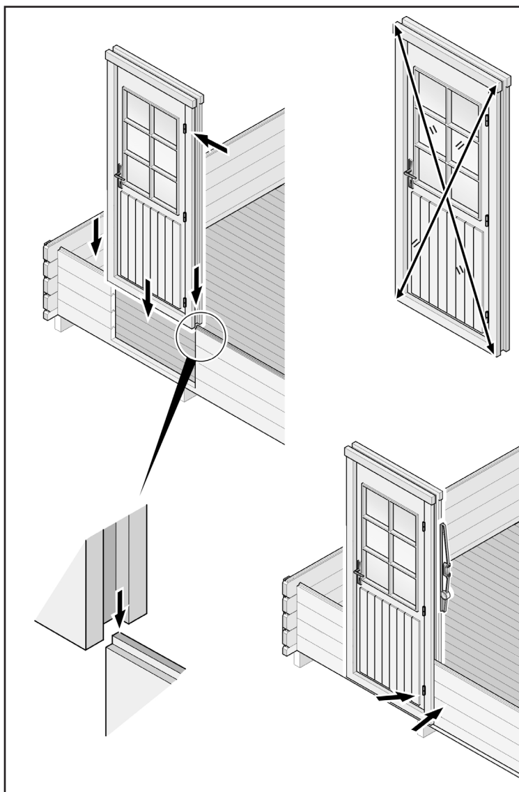
Yleispiirustuksia Allmänna ritningar Allgemeine Zeichnungen Generelle teckningar General drawings Dessins généraux
