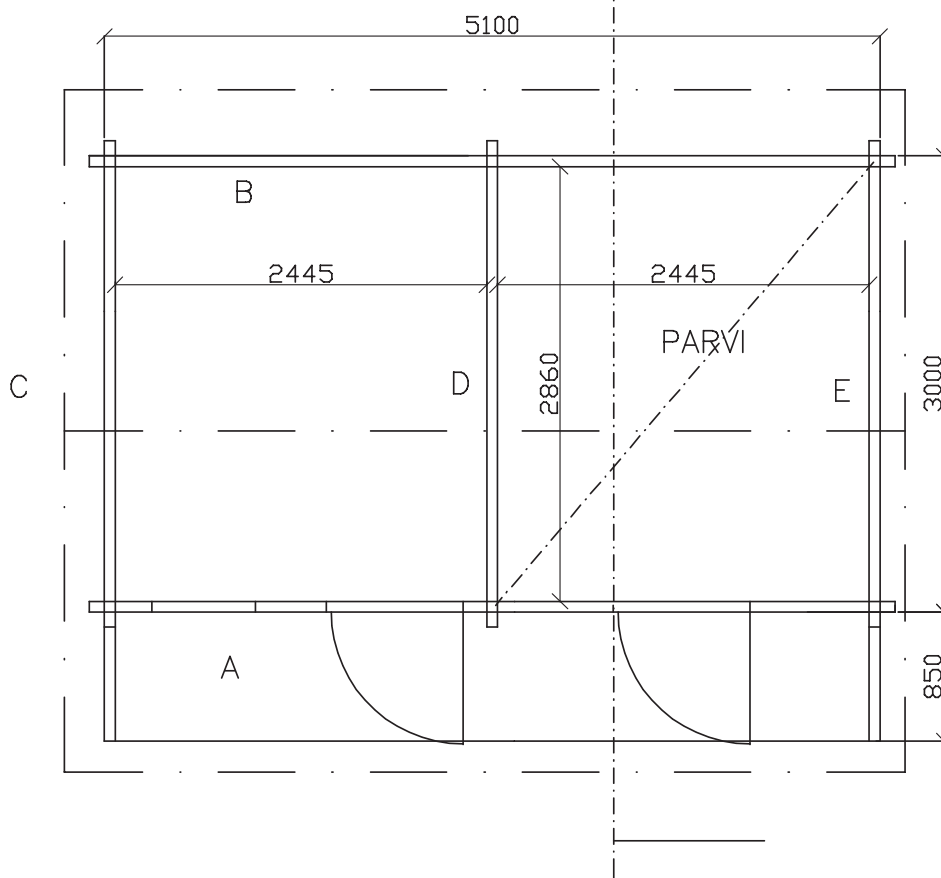
Leikkauskuva
